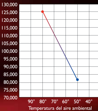
Régimen de calor en BTU por hora UltraTemp 120 & 120 R H/C
