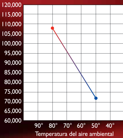
Régimen de calor en BTU por hora UltraTemp 110
